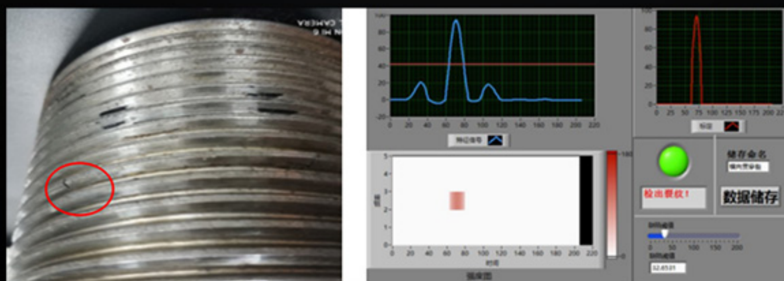
螺纹横向裂纹检测结果
