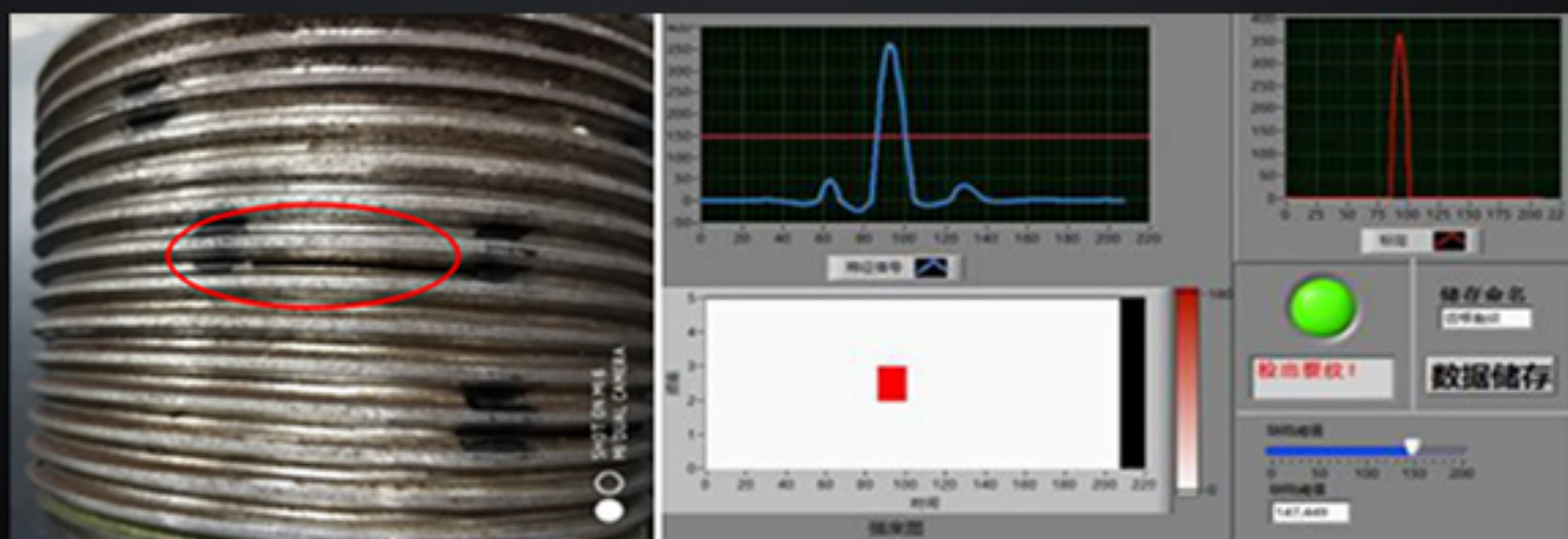
螺纹纵向裂纹检测结果
