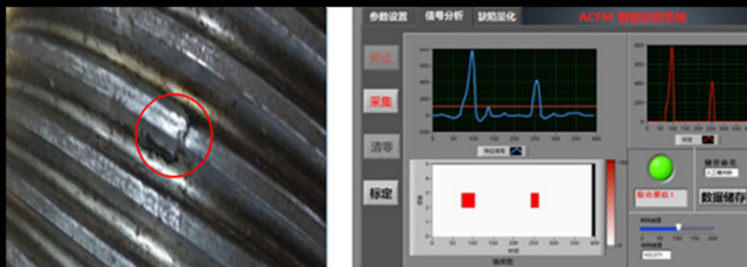
螺纹齿根撕裂检测结果
